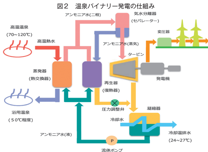
温泉発電(カーリーナサイクル発電)の仕組み
